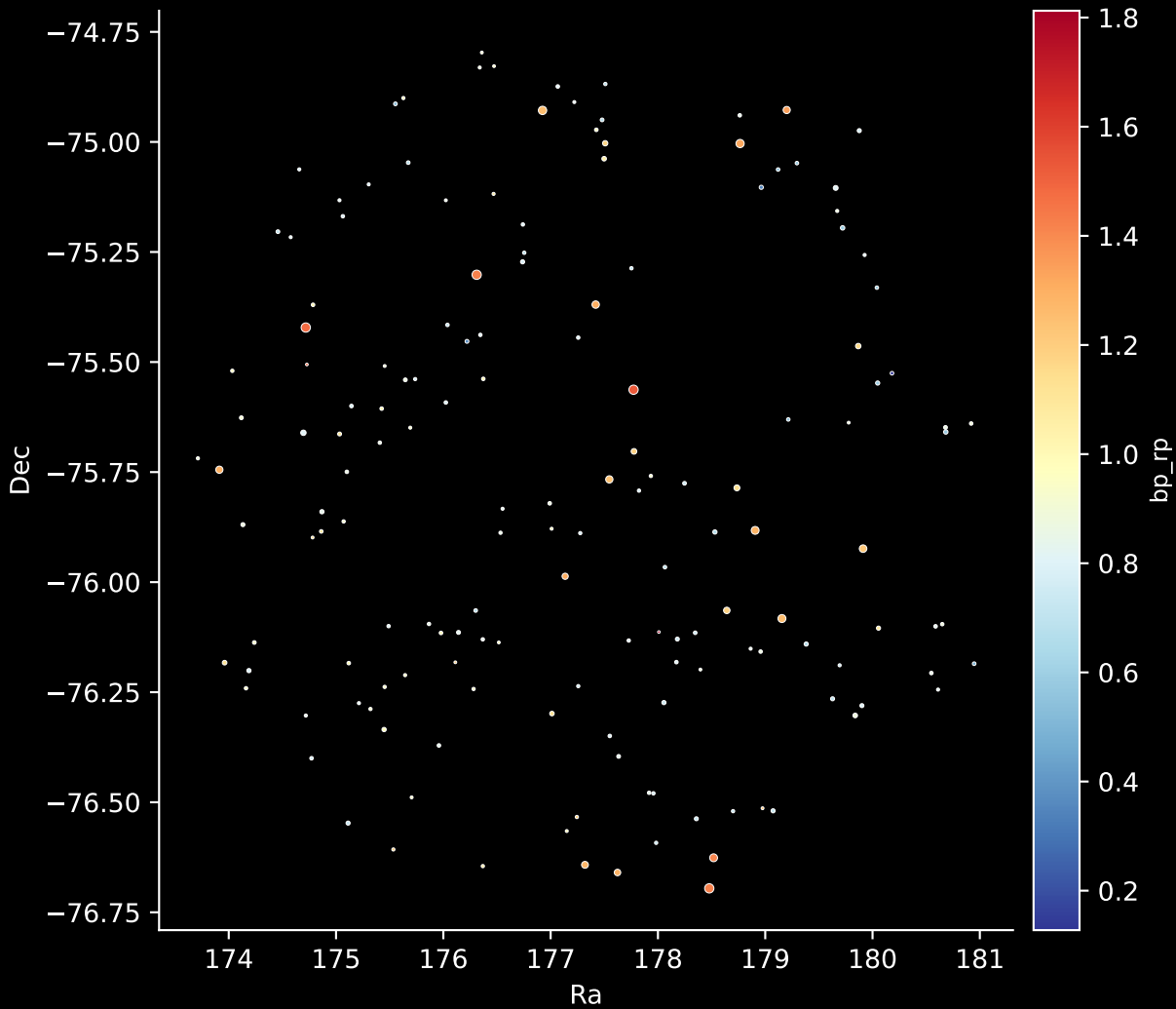
GALAH DR4 Field: [7204] Stars: 158
