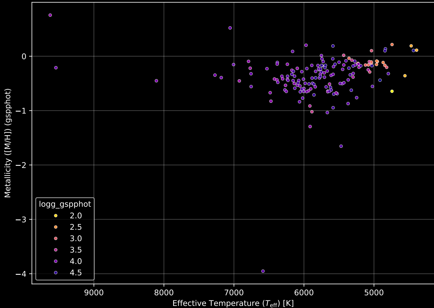
GALAH DR4 Field: [7204] Stellar Population Parameters (n= 158)
